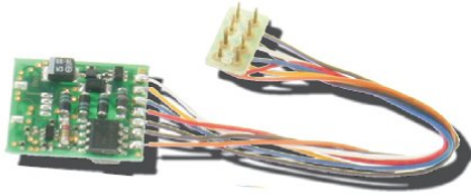
76320 with 8 way NEM 652 Interface Plug
